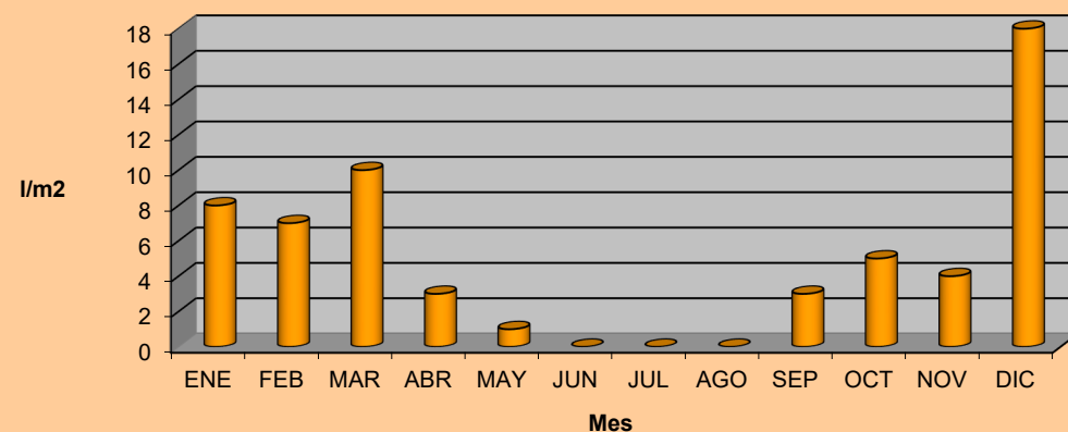
MEDIA MENSUAL DE PRECIPITACIONES MÁXIMAS
