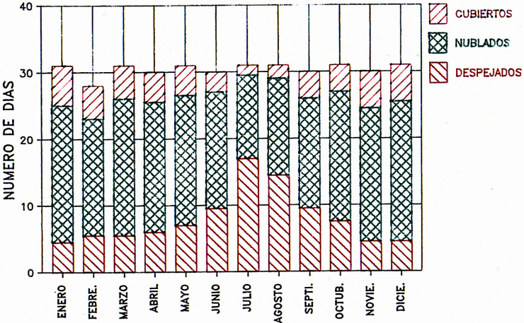
NUBOSIDAD MEDIA MENSUAL FUERTEVENTURA
