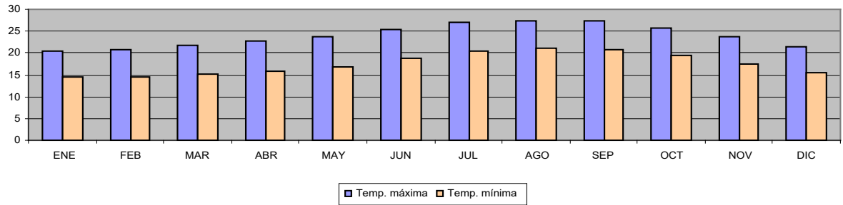
TEMPERATURA MEDIAS MÁXIMAS Y MÍNIMAS
